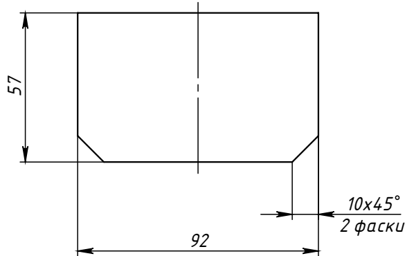
Поз.2 (Ребро)
