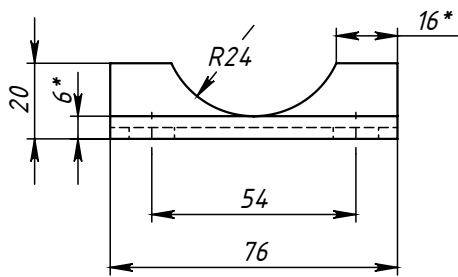
Поз.3 (Ушко) развертка
