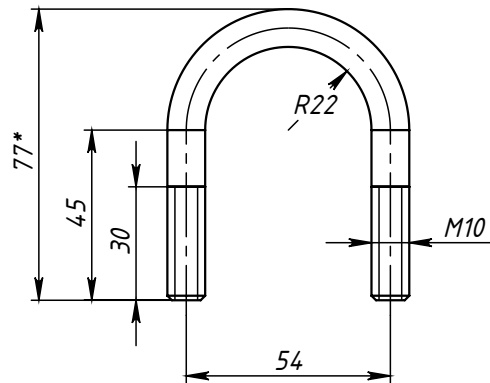
Поз.4 (Хомут)
