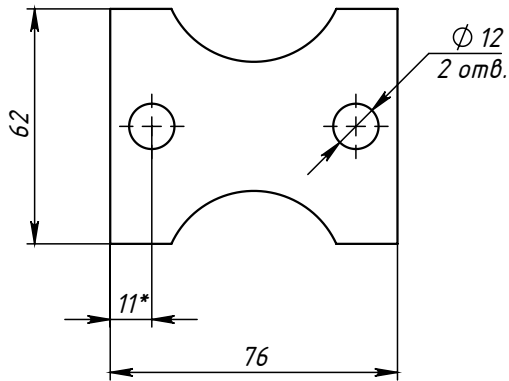
Поз.3 (Ушко) развертка
